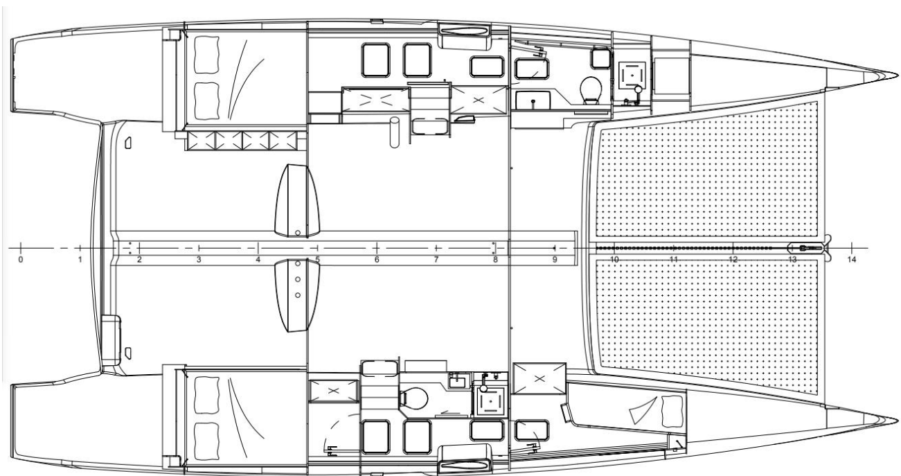
下舱甲板平面图
