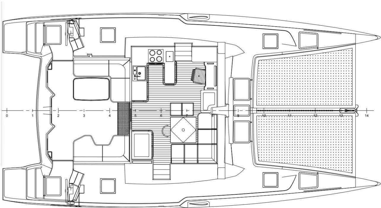
主甲板平面图
